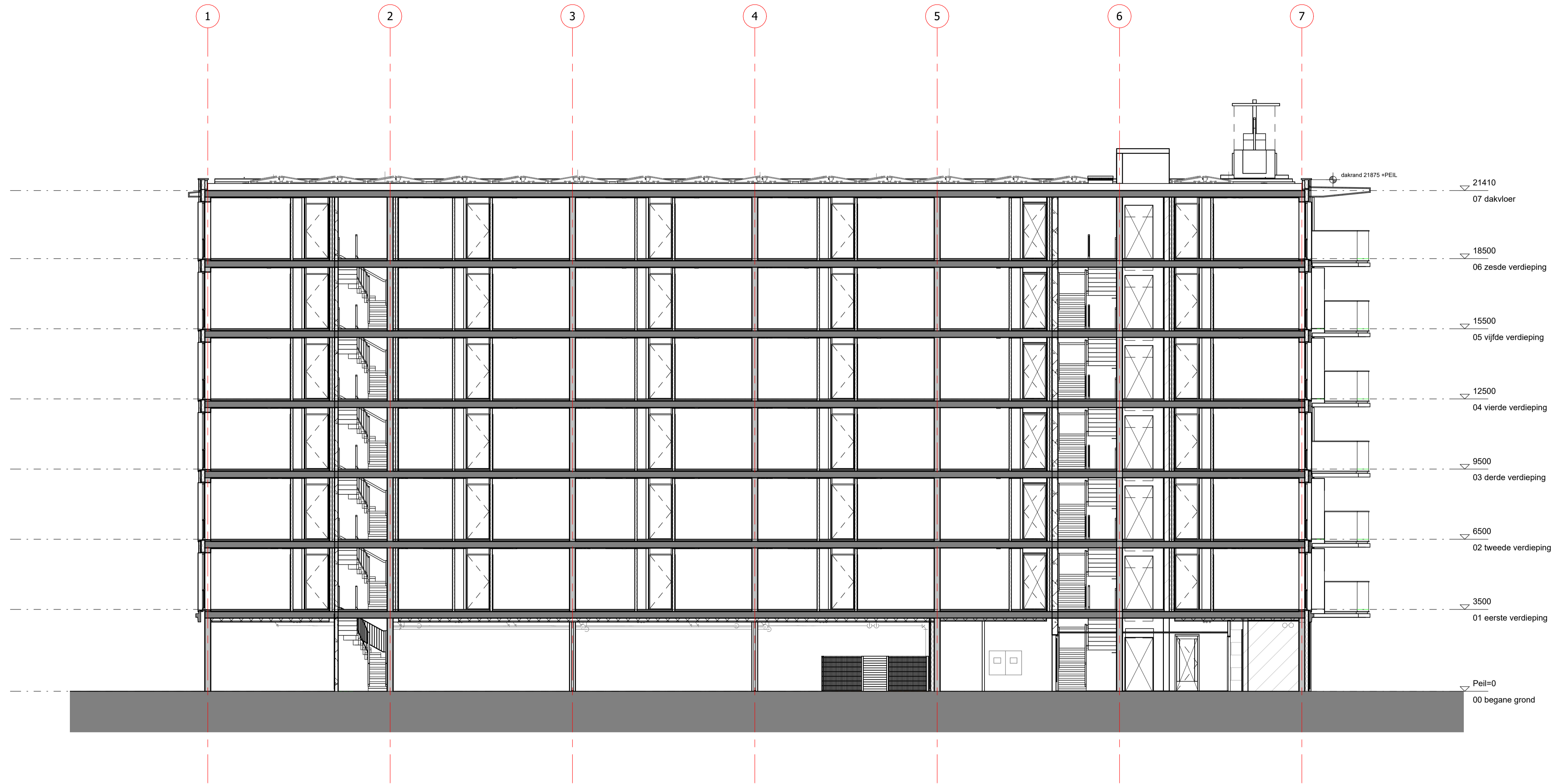
Doorsnede B
