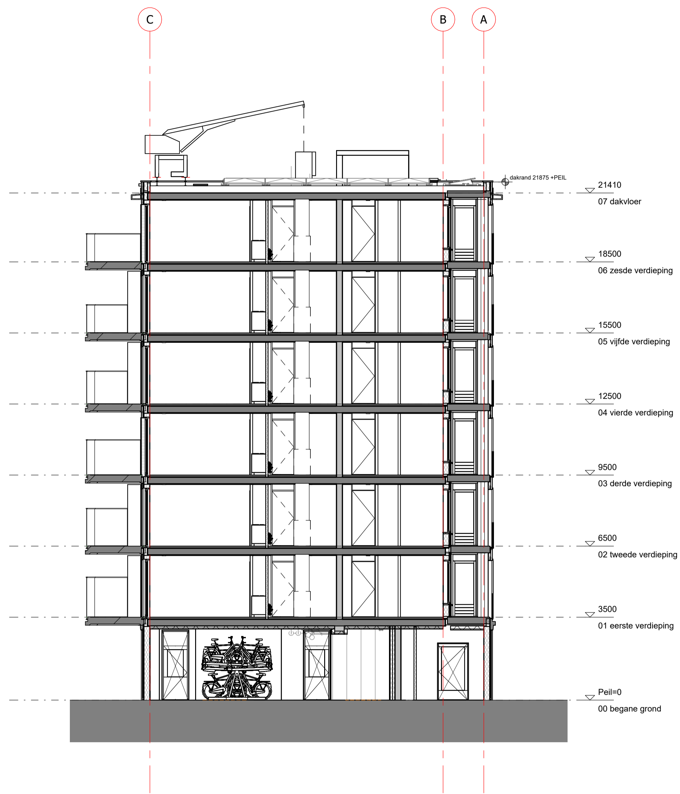
Doorsnede A
